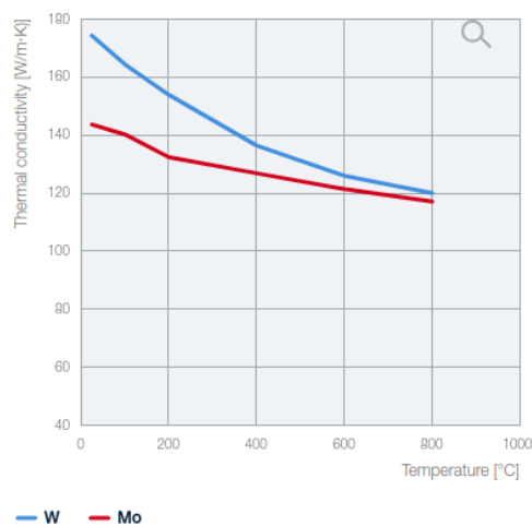
(a) conductividad termina del wolframio y el molibdeno segun la temperatura
