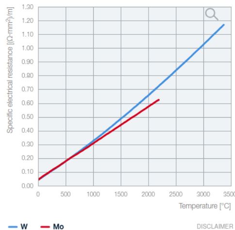
(c) Resistividad electrica del wolframio y el molibdeno segun la temperatura
