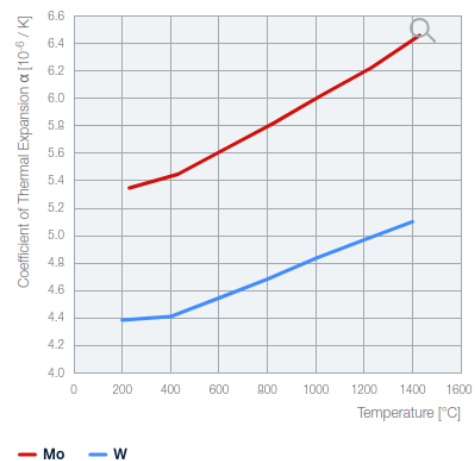
(b) Expansion termina del wolframio y el molibdeno segun la temperatura
